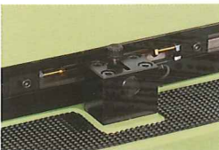
左右切上げ加工装置 Longitudinal stopper
